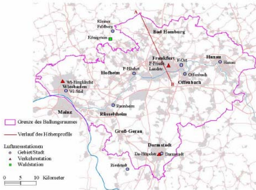
Abbildung 1: Gebiet des Luftreinhalteplanes „Ballungsraum Rhein-Main“
