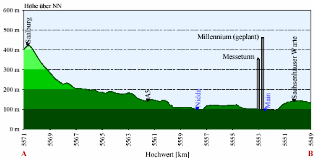
Abbildung 3: Geländeschnitt von der Saalburg zur Sachsenhäuser Warte
